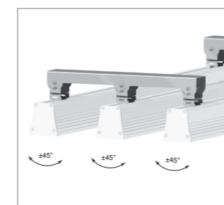
Uchwyty 3x do montażu 3 opraw Handle 3x for suspension of 3 luminaires
